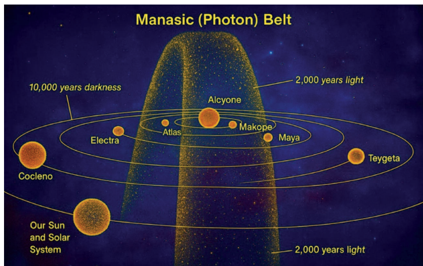
Abb. 3: Der Photonenring
